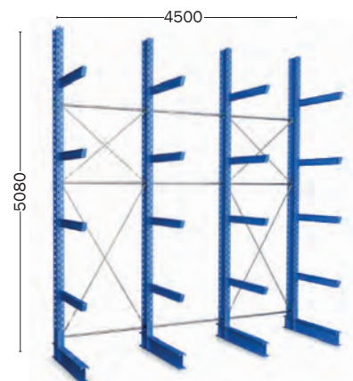
Esimerkki 2 1-puoleinen, 4-pylvästä Jalka + 4 uloketasoa Korkeus 5080 mm (pylväs IPE240)
