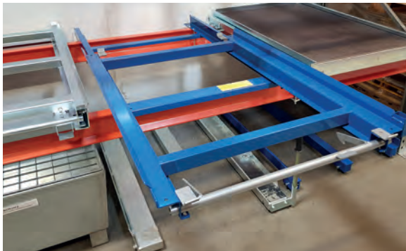
1. Vetotaso vaakapalkille, maalattu.
