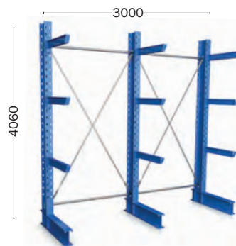
Esimerkki 1 1-puoleinen, 3-pylvästä Jalka + 3 uloketasoa Korkeus 4060 mm (pylväs IPE220)
